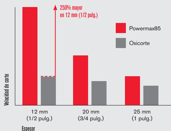
Rendimiento de corte relativo, acero al carbono
